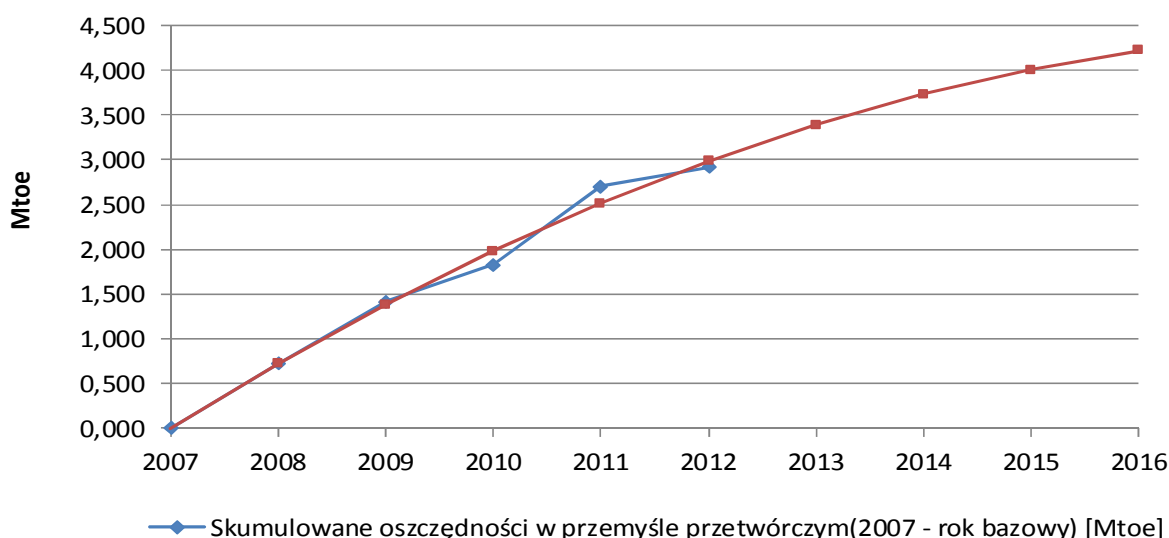
Rys. 8 Oszczędności energii w przemyśle przetwórczym [Mtoe] oraz aproksymacja kwadratowa w latach 2007-2016
